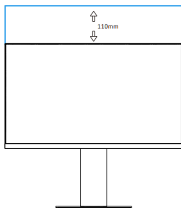
Regolazione dell'altezza della testa del monitor: 0-110 mm
